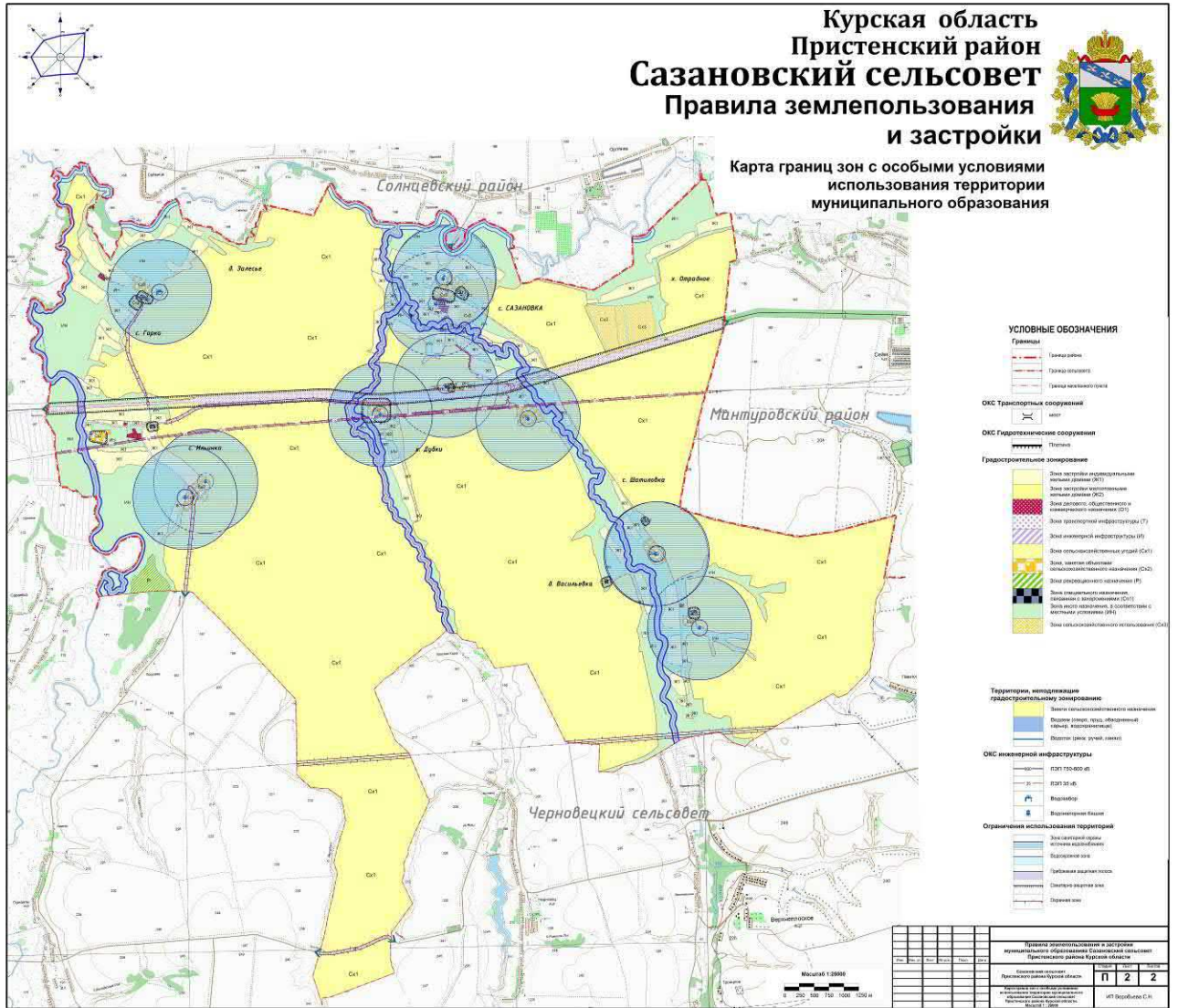
Рис.2. Карта границ зон с особыми условиями использования территории муниципального образования «Сазановский сельсовет» Пристенского района Курской области
