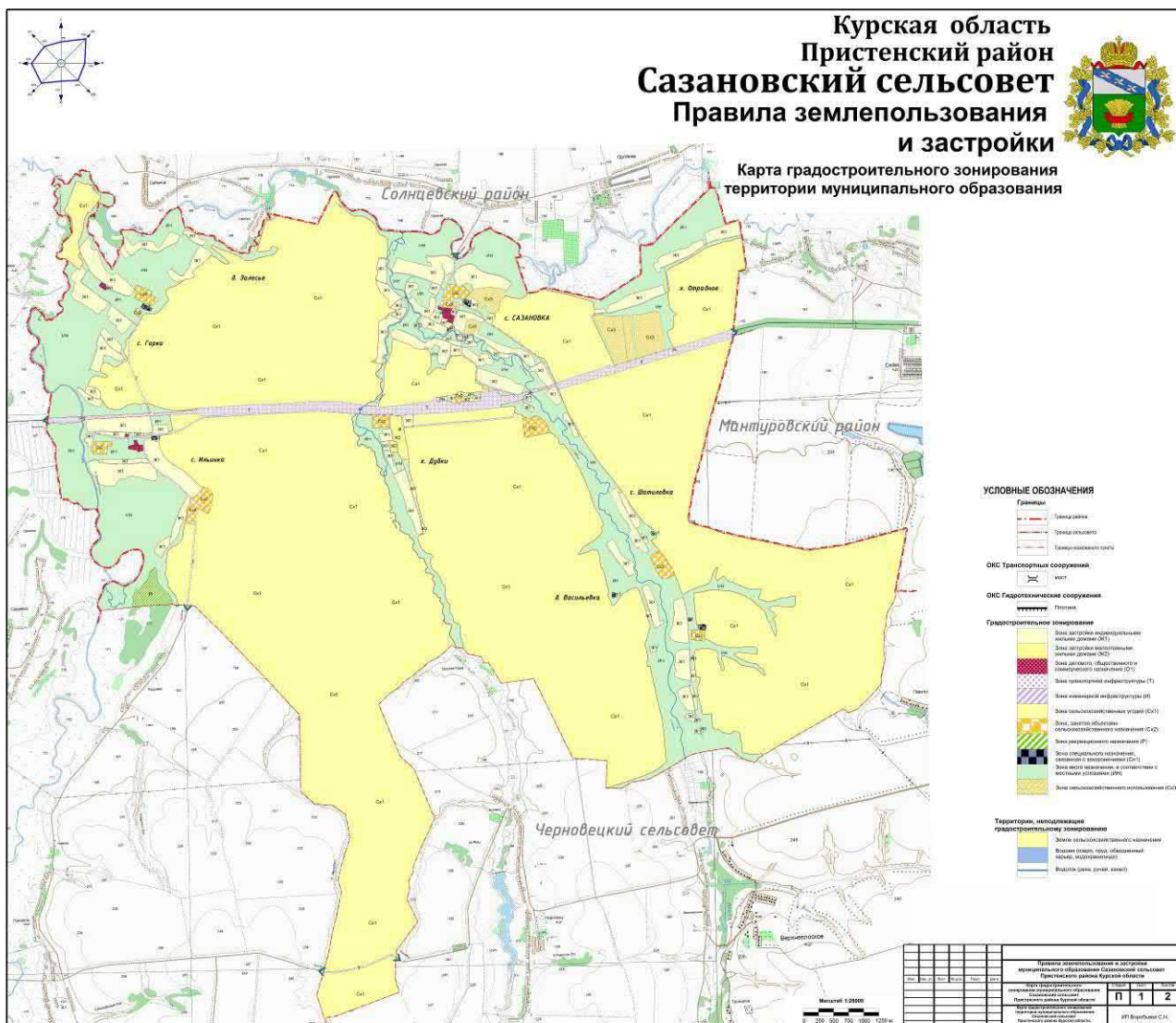
Рис.1. Карта градостроительного зонирования территории муниципального образования «Сазановский сельсовет» Пристенского района Курской области
